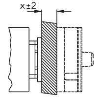
LS... +VW“x“ Verlängerte Schalterwelle
