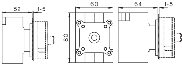
LS16 E.., LS25 E.., LS32 E.., ..A2 ..A2+2, ..A4.
