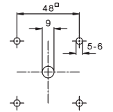
Bohrplan Montageschraube S3631N M=1,2-1,4 Nm
